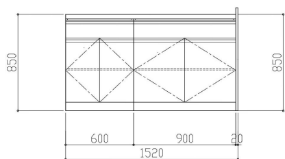
展開A図
